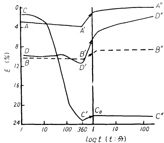
マツ材切線方向圧縮 ( 20\text{kp/cm}^2 ) A A' A'' : 湿潤状態 B B' B'' : 全乾状態 C C' : 湿潤—全乾 (360分) C' C'' : 全乾状態 D D' : 全乾—湿潤 (360分) D' D'' : 湿潤状態
