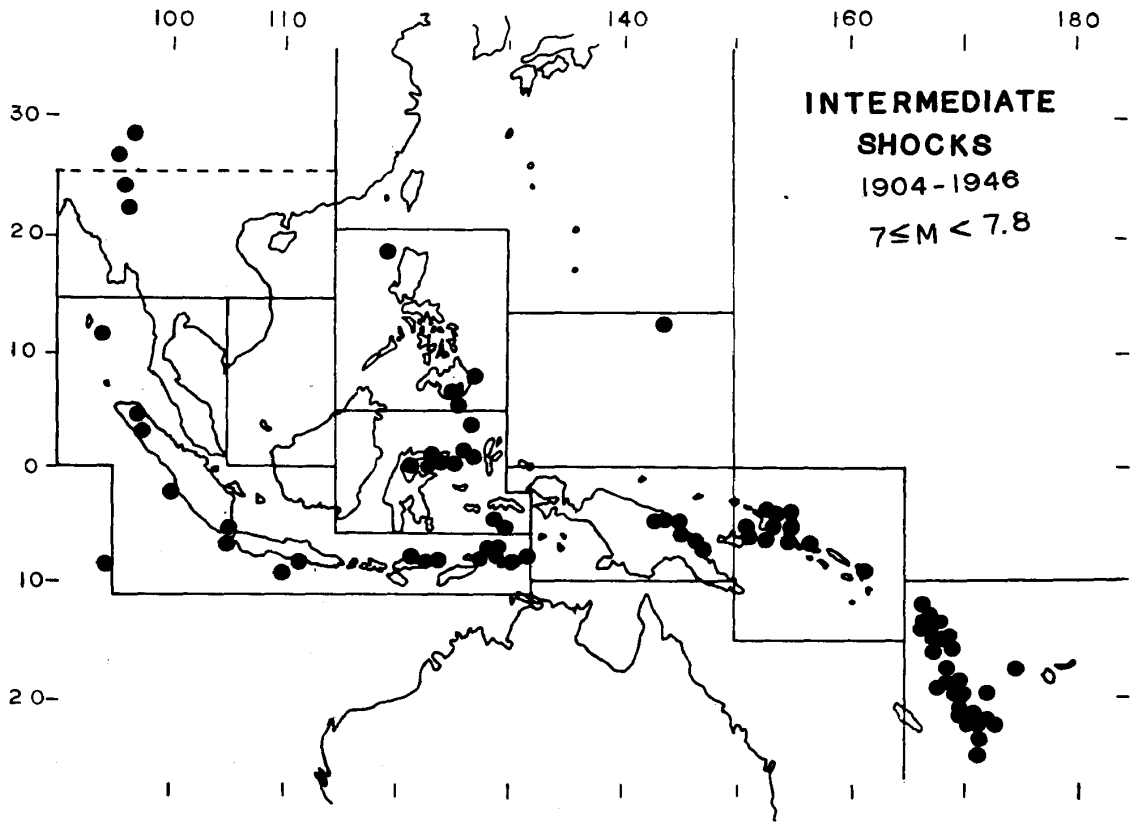
第 6 图 中深大地震分布图 (1904—1946)
