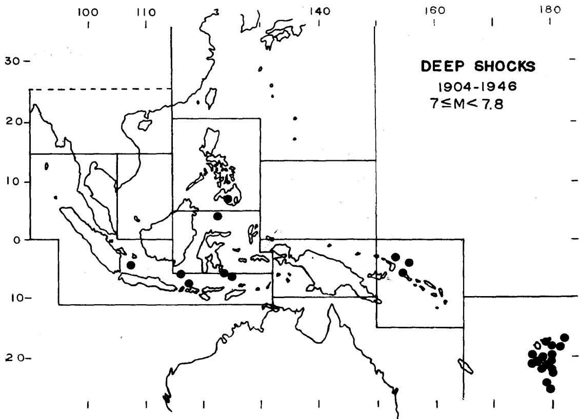
第 7 图 深発大地震分布图 (1904—1946)
