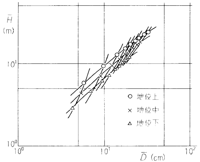
図9 時間方向と要因方向の相対生長関係 各時点ごとに地位の差による相対生長関係と地位ごとに時間の差による相対生長関係はことなる。(林分収穫表 24) による。)
