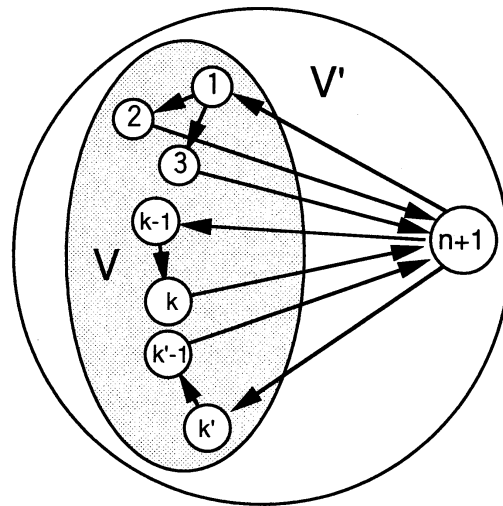
図4. 補題2.3の証明
