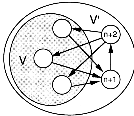
図3. 補題2.2の証明
