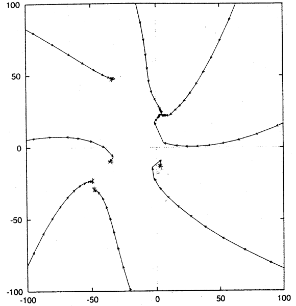
図 40. P_{32} に対する SOR 反復 ( \omega = 1.0 )
