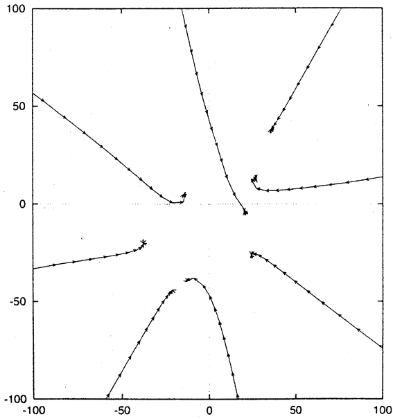
図 27. P_{14} に対する D-K 反復
