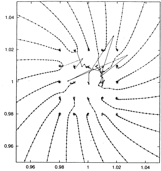
图 18. SOR (1.7), \omega = 1.0 (放大图).
