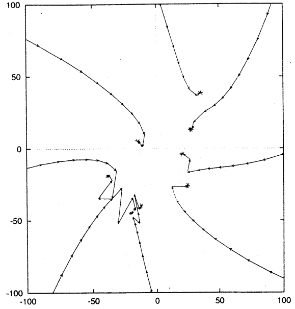
図 28. P_{14} に対する SOR 反復 ( \omega = 1.0 )
