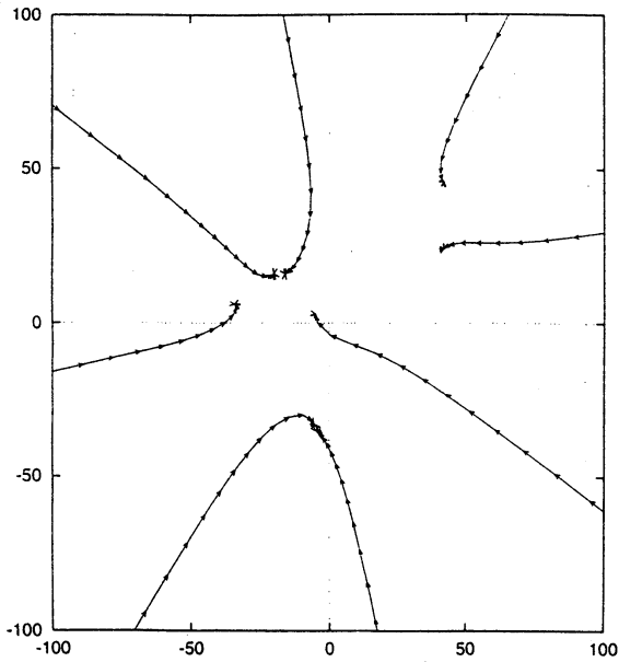
図 25. P_{13} に対する D-K 反復
