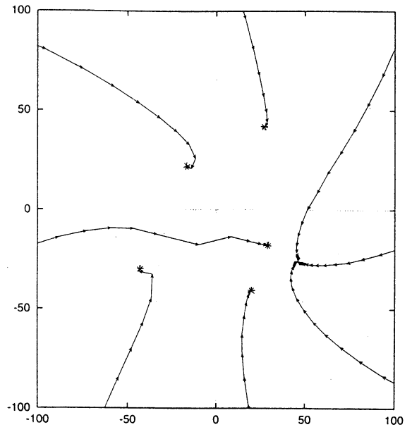
図 42. P_{33} に対する SOR 反復 ( \omega = 1.0 )
