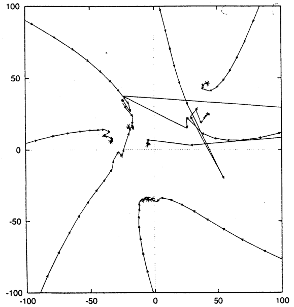
図 26. P_{13} に対する SOR 反復 ( \omega = 1.0 )
