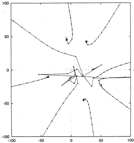
図 31. P_{22} に対する D-K 反復
