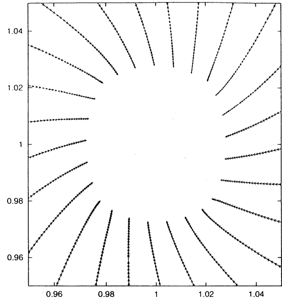
图 10. SOR (1.6), \omega = 0.6 (放大图).
