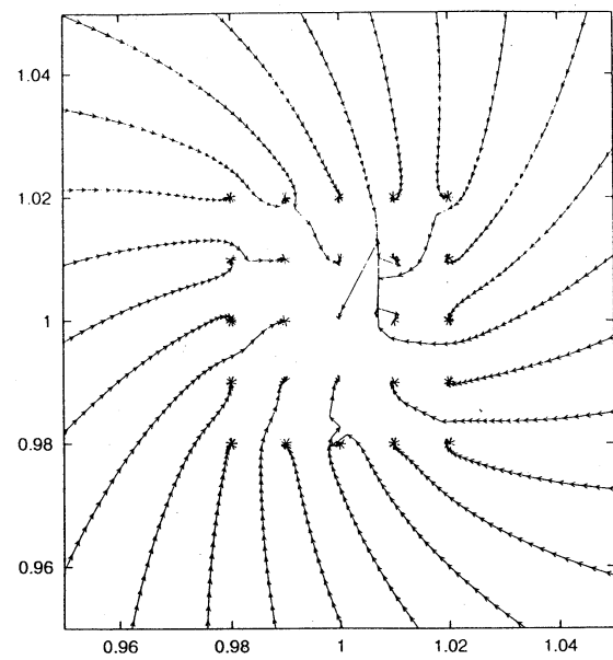
图 12. SOR (1.6), \omega = 1.0 (放大图).
