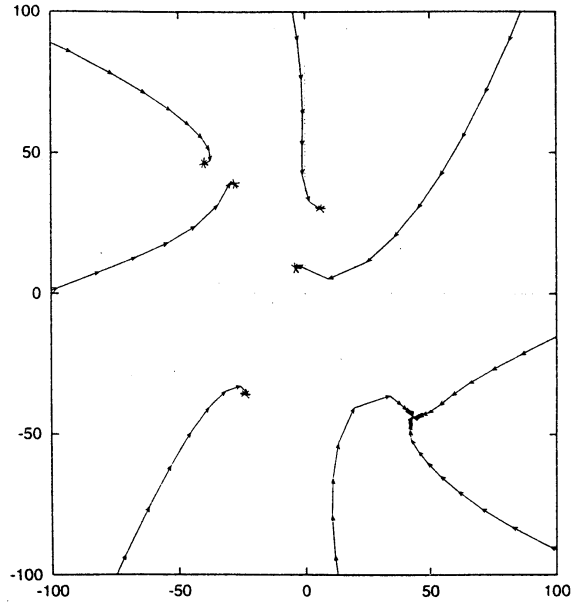
図 38. P_{31} に対する SOR 反復 ( \omega = 1.0 )
