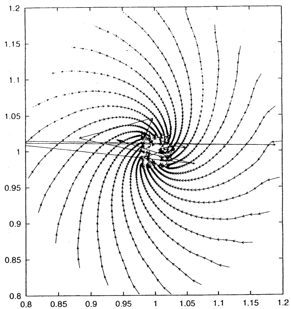
图 15. SOR (1.6), \omega = 2.0 .
