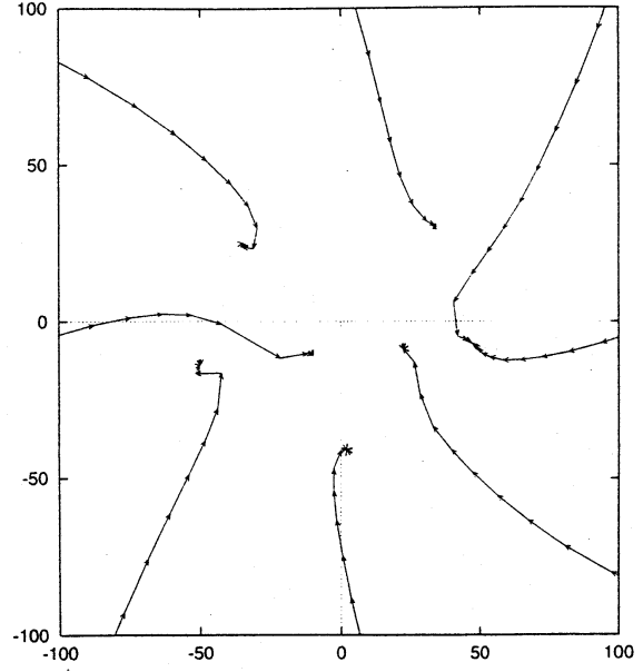
図 36. P_{24} に対する SOR 反復 ( \omega = 1.0 )
