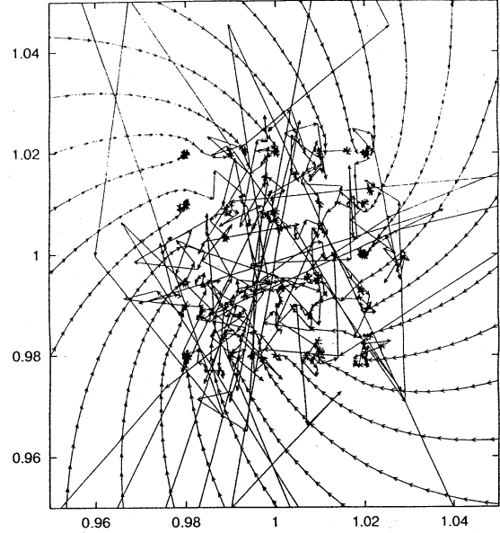
图 14. SOR (1.6), \omega = 1.8 (放大图).
