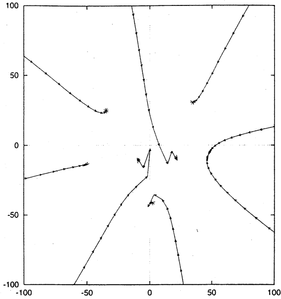
図 35. P_{24} に対する D-K 反復
