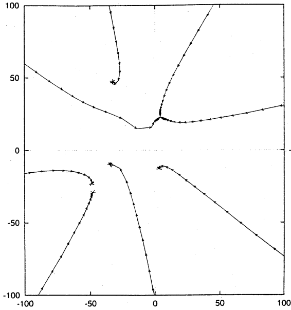
図 39. P_{32} に対する D-K 反復
