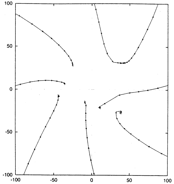
図 30. P_{21} に対する SOR 反復 ( \omega = 1.0 )
