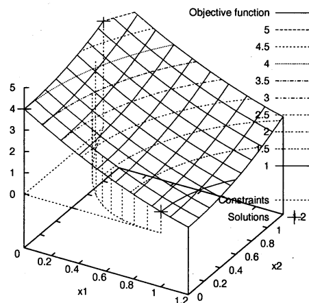
Fig. 2. 例題 2. 目的関数と制約集合
