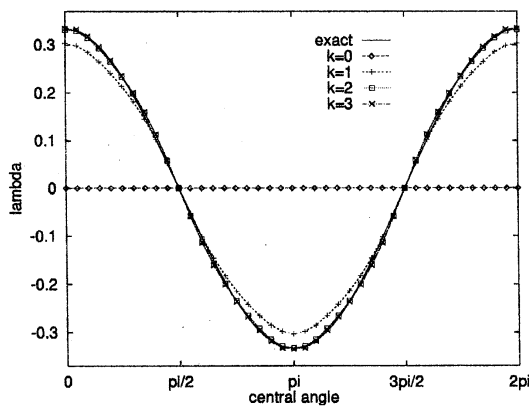
図 9: \lambda^{(k)} と \lambda(\lambda^{(0)} = 0)
