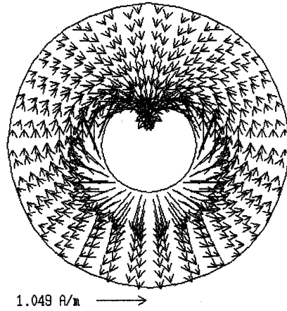
図 8: 数値解 H_0^{(4)}
