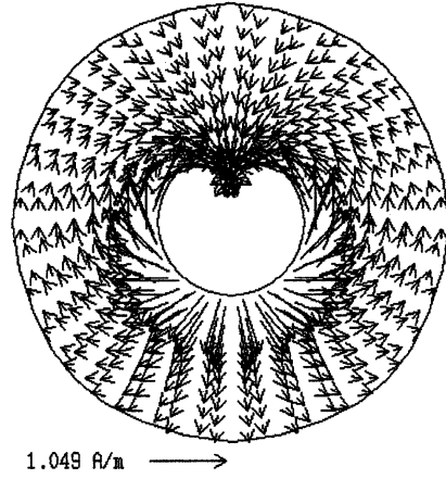
図 6: 真の解 H
