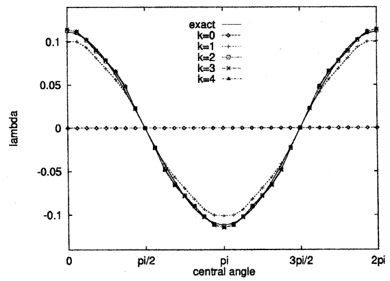
図 10: \lambda^{(k)} と \lambda(\lambda^{(0)} = 0)
