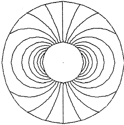
図 5: 真の解 u
