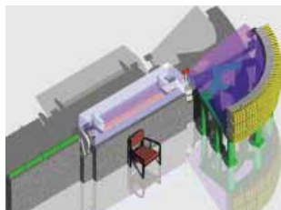
MEIZE型中性子散乱装置の完成予想図
