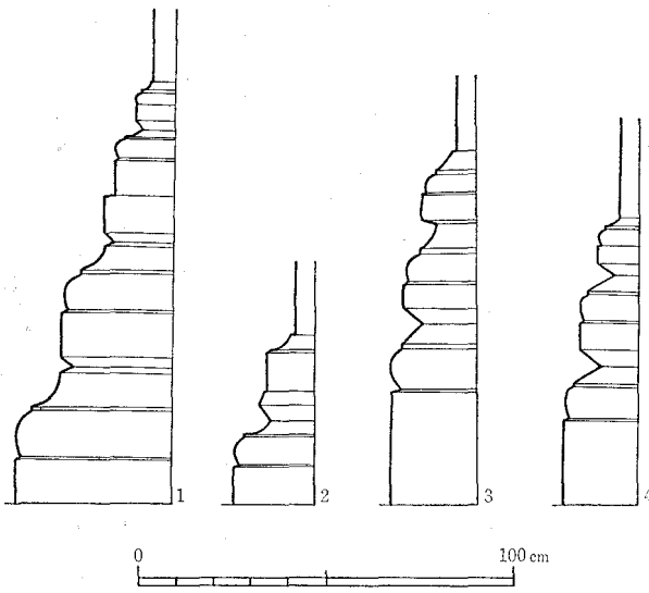
挿圖 2 ハツダ佛塔刳型の種類 1. タパカラーンNo141大塔 2. タパカラーンNo33塔 3. ラルマ主塔 4. タパシヨトル主塔
