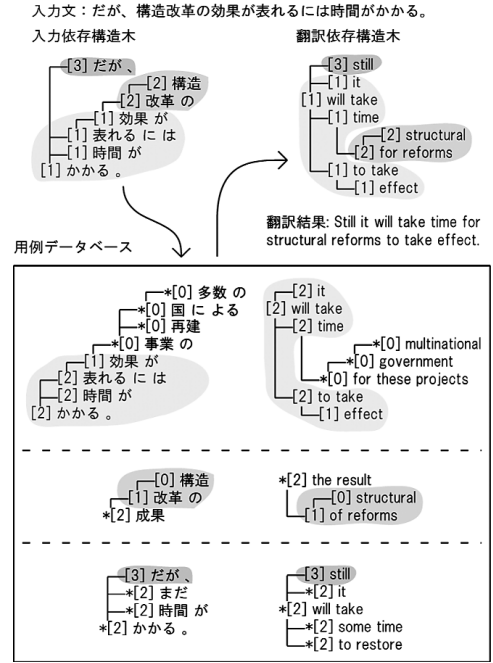
図1. 用例ベース機械翻訳例
