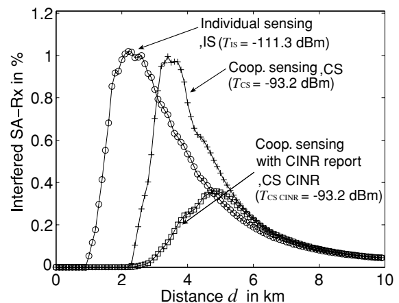
図2. 検出情報の交換 (Coop. sensing with CINR report) によってSA-Rxへの干渉が大幅に低減できる
