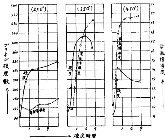
第六圖 Be-Cu 合金 (2.5% Be) の焼戻の相違に 依る電気傳導度並に硬度の變化
