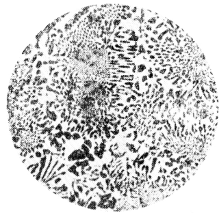
第十九圖 Be-Si 共晶組織 (倍率 150)
