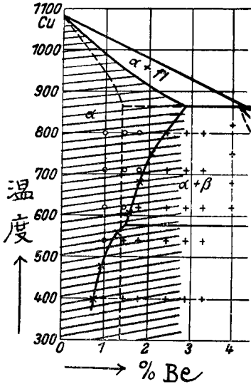
第三圖 Be-Cu 合金の状態圖
