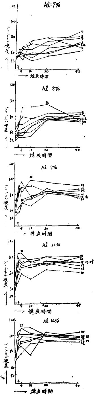
第4圖 200°C 燒灰硬化曲線圖
