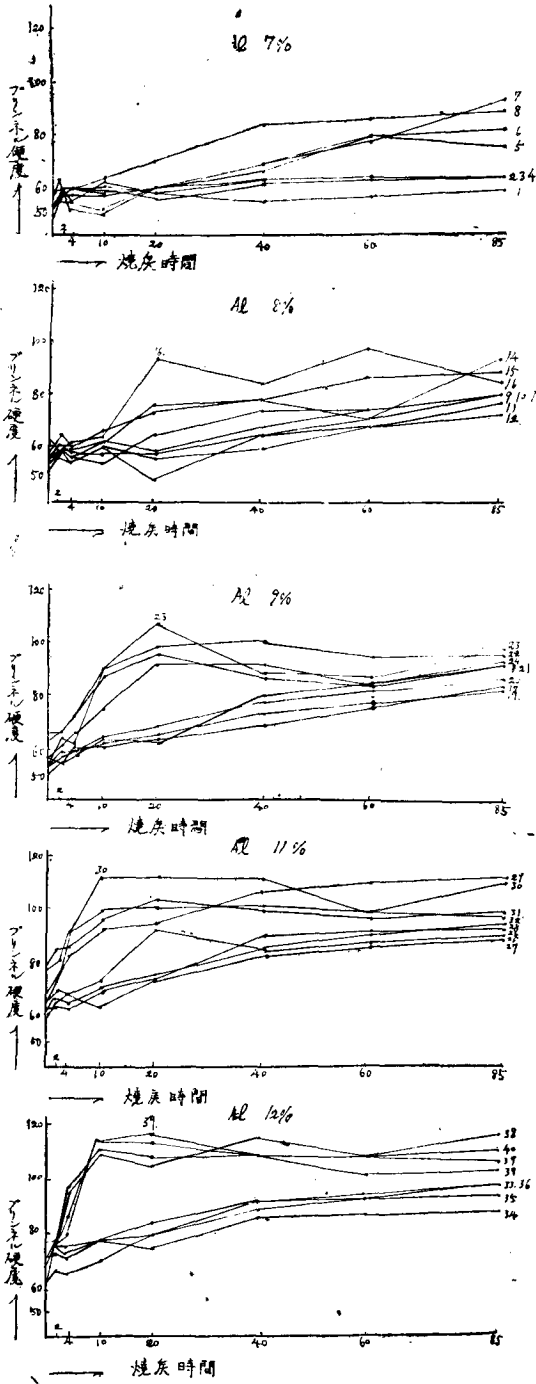
第3圖 150°C 燒灰硬化曲線圖
