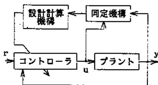
図1. 2 STRの構成概要
