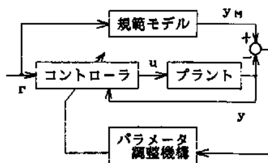
図 1. 1 MRACS の構成概要
