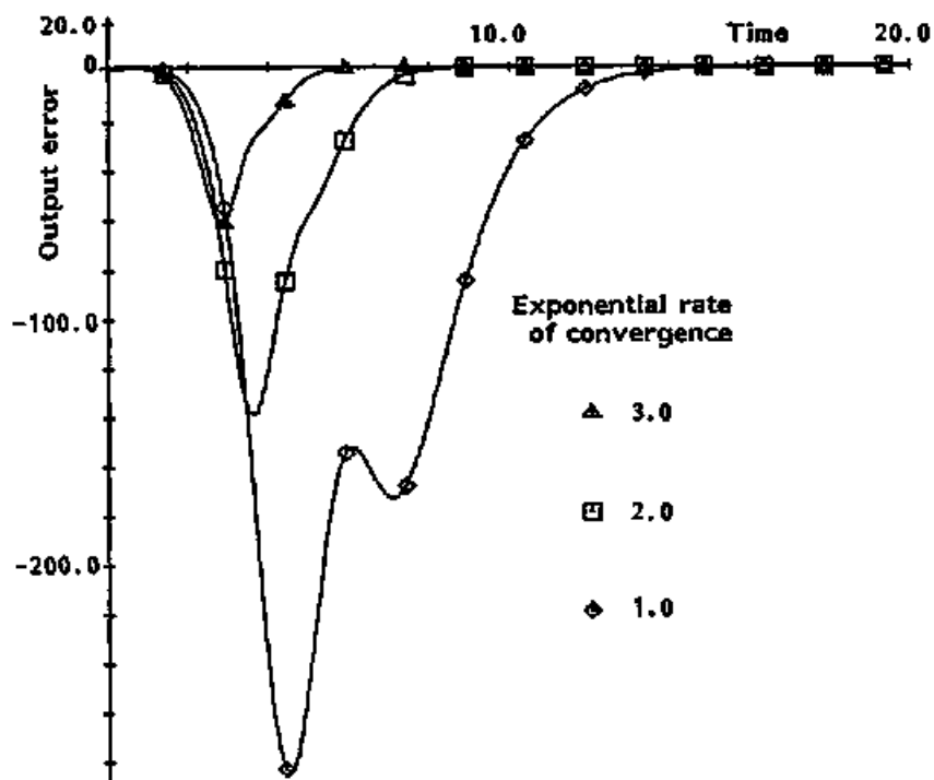
図 2. 3 基本構成のMRACSの出力誤差
