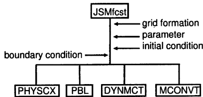
Fig. 2 Structure of JSM
