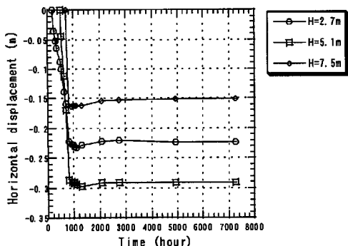
Fig. 4 Horizontal displacement
