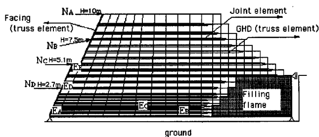
Fig. 7 FEM mesh
