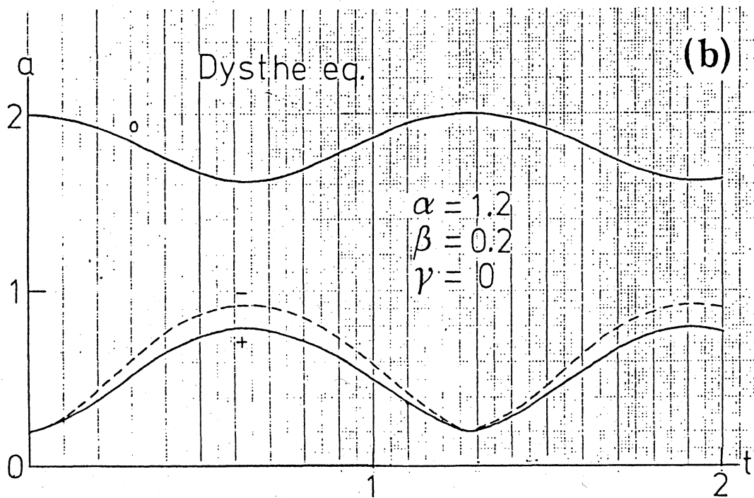
図1. (3.4)~(3.7)の数值解。(初期値: a_0=2 , a_1=a_2=0.2 )
