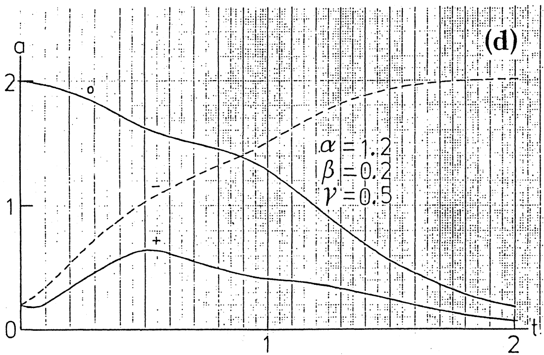
図1. 非線形散逸項を含む場合 ( \sigma \neq 0 ) (+: 高側帯波、 -: 低側帯波) (c) \gamma = 0.2 : 非対称、非回帰 (d) \gamma = 0.5 : 非対称、非回帰
