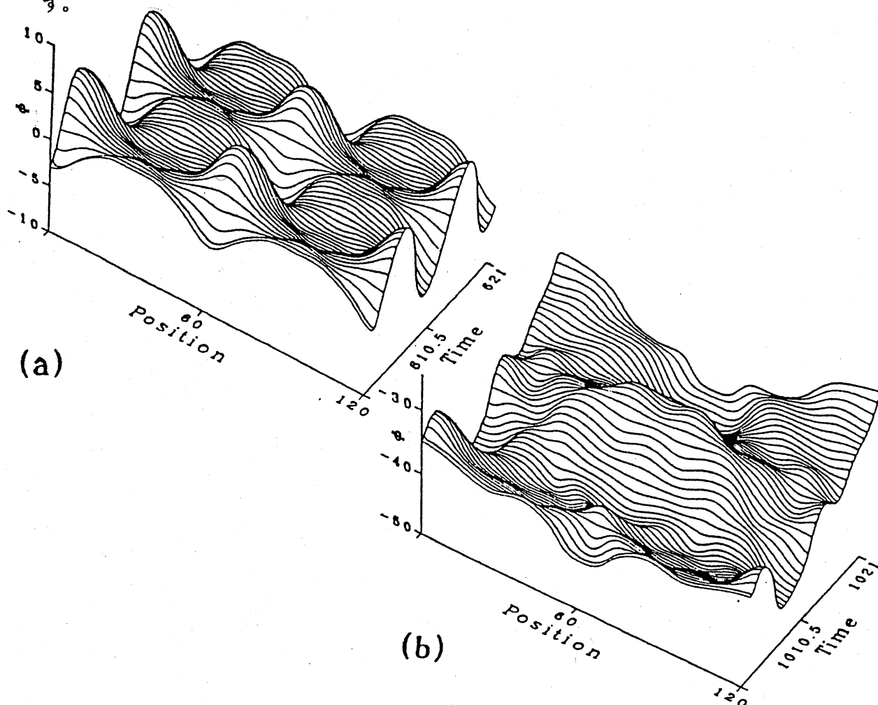
図2. SG方程式: \phi_{tt} - \phi_{xx} + \sin \phi = \gamma \sin \omega t - \varepsilon \phi_t の数値解 (\varepsilon = 0.2, \omega = 0.6) (a) 周期的発展 ( \gamma = 0.8 ) (b) カオスの発展 ( \gamma = 1.0 )
