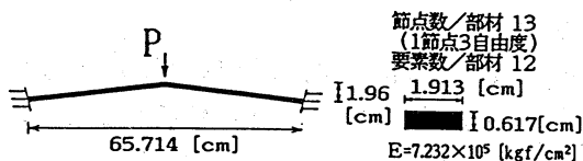
図-1 2本の部材で構成される山型はりの問題
