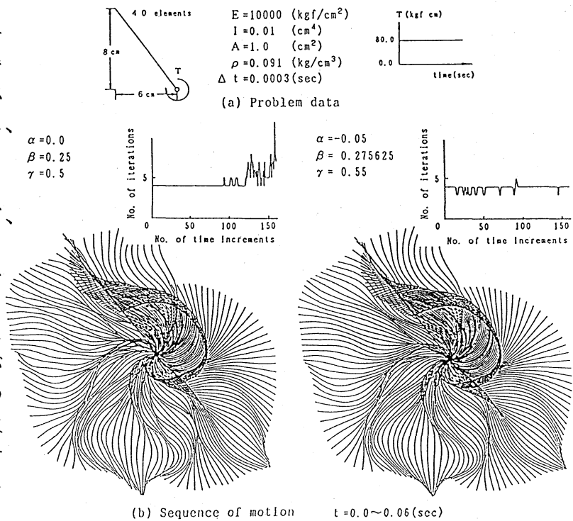
図-11 端部にトルクを受けて回転する柔らかい棒の解析例
