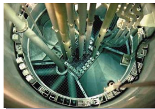
研究用原子炉KURの炉心
