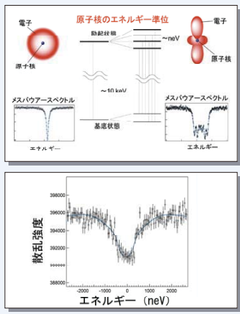
図1. 原子核のエネルギー準位と電子状態の関係。原子核のエネルギー準位(状態)が原子核の周りの電子の状態の違いを反映して変化します(ここでは準位が分裂する様子を表しています)。このとき、このエネルギー準位の変化を反映してメスバウアー分光法も異なるものとなります。 図2. ^{73}\text{Ge} 放射光メスバウアー吸収スペクトル(励起エネルギー: 68.752 keV)測定試料にはグルマニウム酸リチウム( \text{Li}_2\text{GeO}_4 )を用い、基準試料としてはGe酸化物( \text{GeO}_2 )を用いました。
