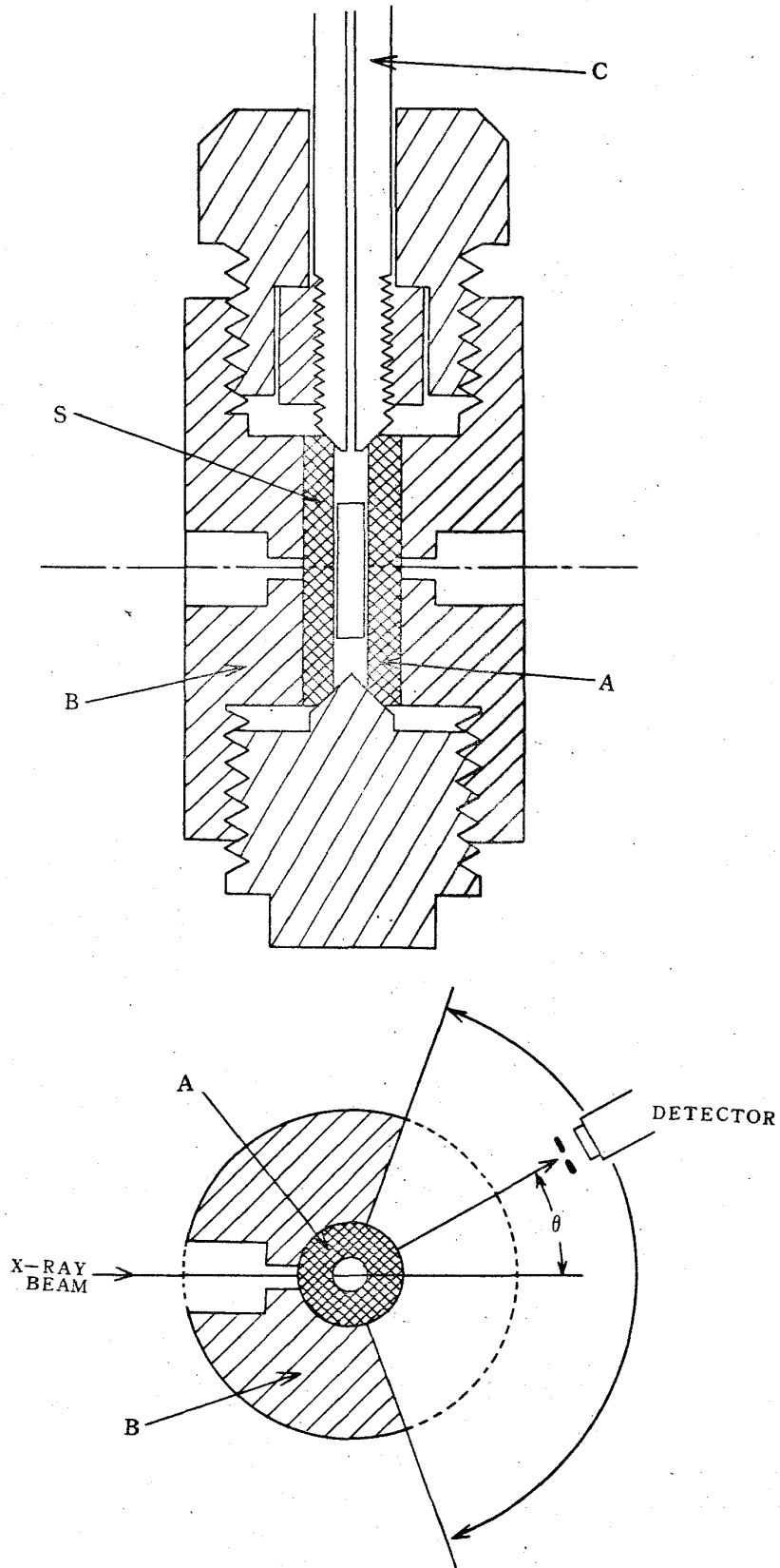
図 1. 装置の略図
