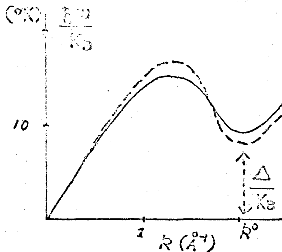
第1図 He 4 の縦波（実線は実験値）
