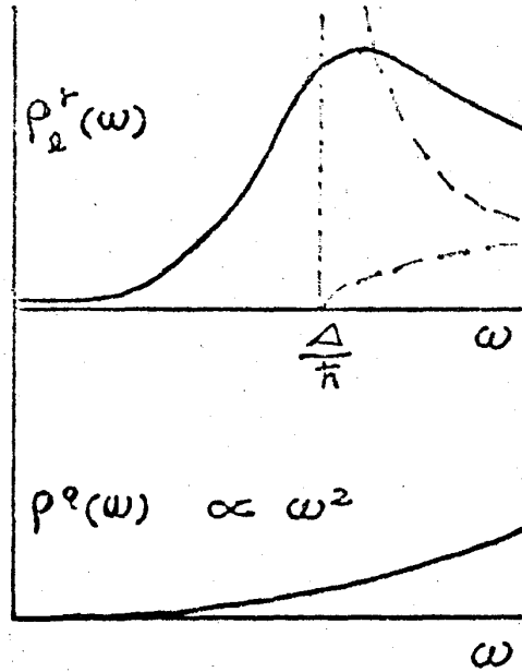
第5図 \rho_l^\Gamma(\omega) の概形
