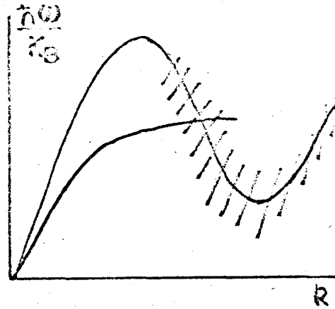
第4図 不定形固体のフォノンの概念図
