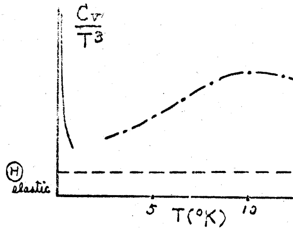
第3図 不定形 SiO 2 の比熱
