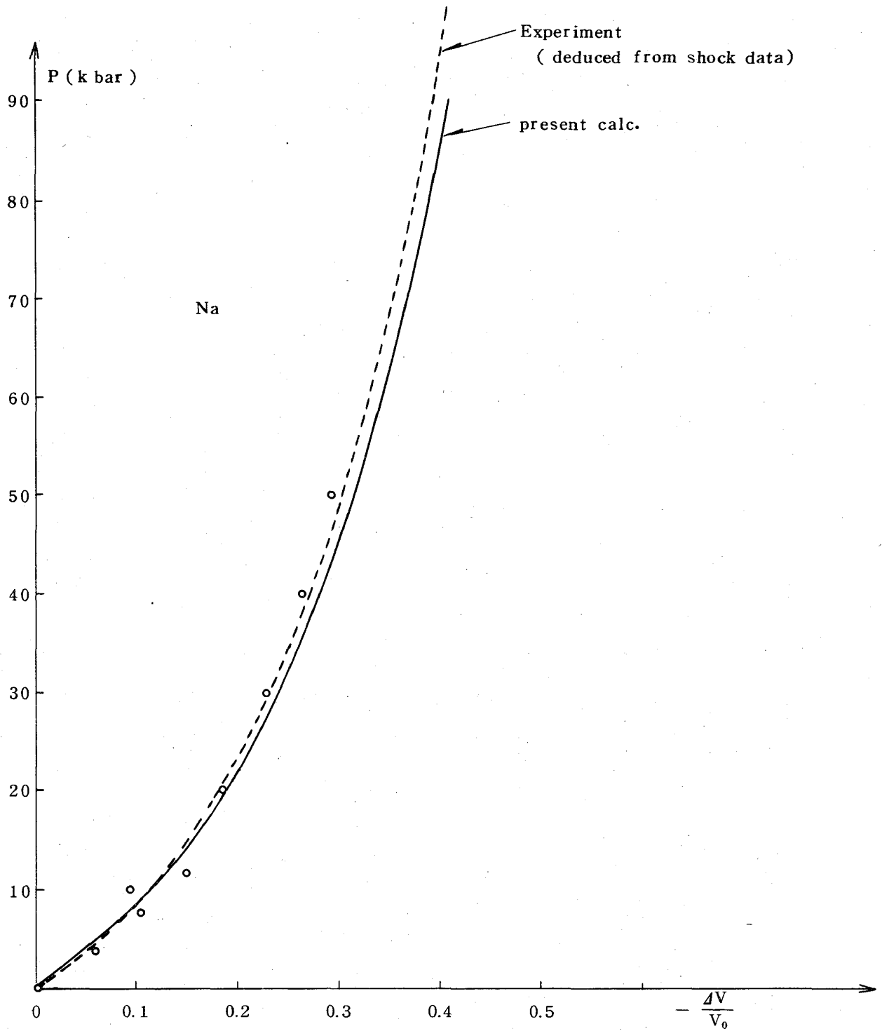
図 2 擬ポテンシアル・モデルから得られる状態方程式 ( T=0, \text{Na} )。実線は計算値, \circ は Bridgman の実験値, 点線は shock wave による実験値。図 3~7 も同じ。
