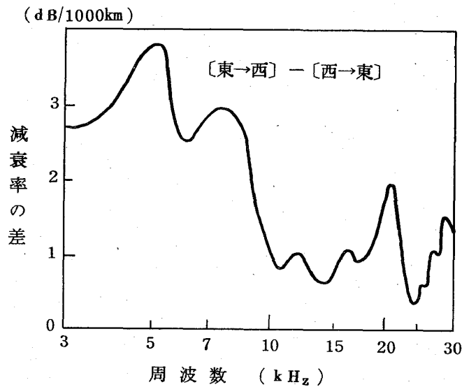
図1. 東→西伝播と西→東伝播の減衰率の差の周波数依存性 (Taylor, 1960)。雷放電に源を発生し、地表と電離層下端の間を伝わる空電の波形観測から得られたもの。東→西伝播の方が減衰されやすいことを示している。
