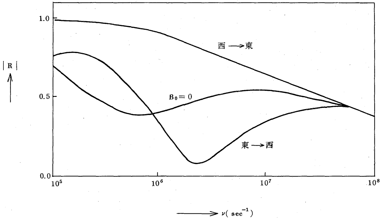
図 6-a 反射係数の衝突回数による変化 (Barber et al, 1959)。 \omega = 10^5/\text{sec} , \Omega_e = 5 \times 10^6/\text{sec} , \pi_e = 10^6/\text{sec} , \theta_i = 78.5^\circ ととっている。
