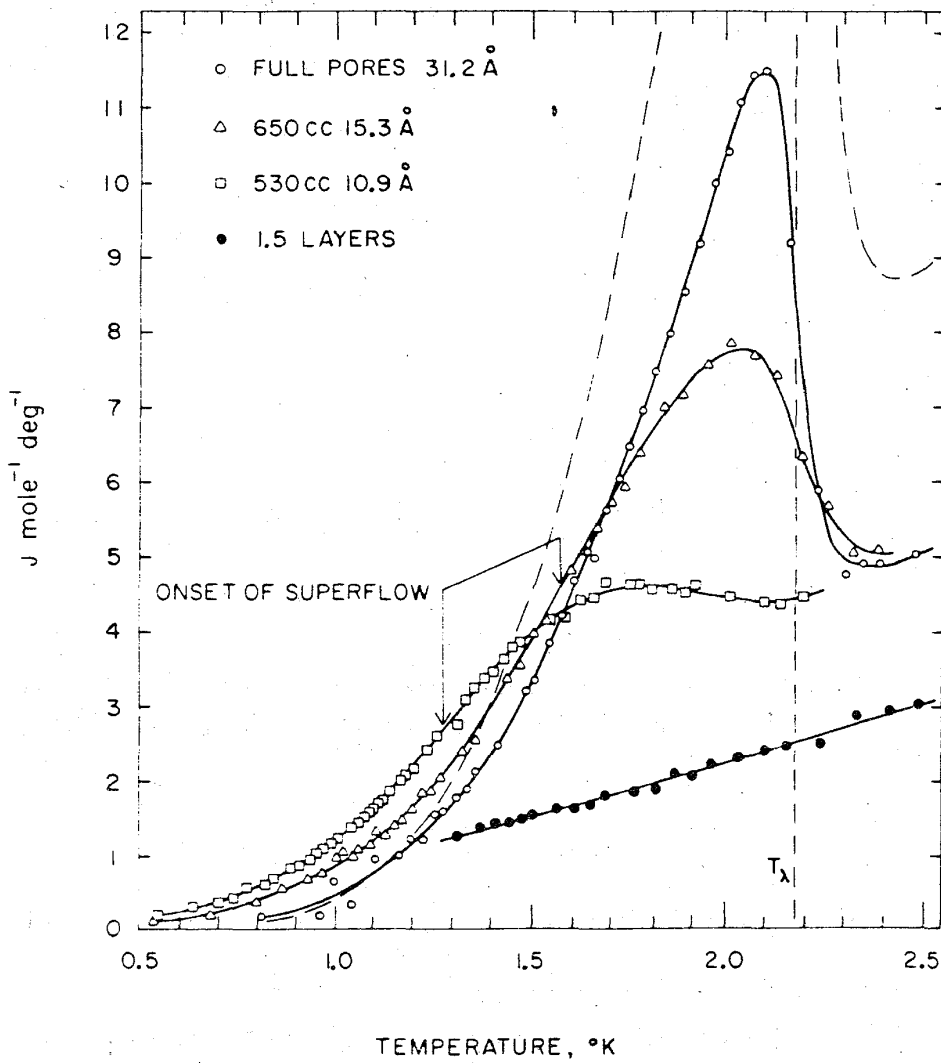
第3図 Multilayer specific heat of He 4 adsorbed on Vycor. (Brewer 1) による)
