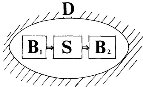
(図4) 2つの熱浴 B_1, B_2 と散逸的熱浴 D
