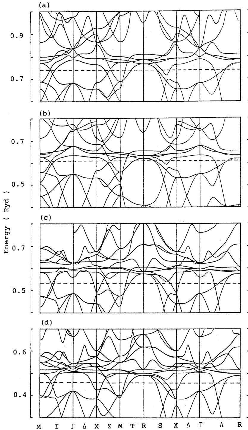
図1. LSD 近似の交換・相関相互作用に基づく、フエルミ・エネルギー 近傍の APW エネルギー・バンド構造。 (a) USi_3 , (b) UGe_3 , (c) USn_3 , (d) UPb_3 .
