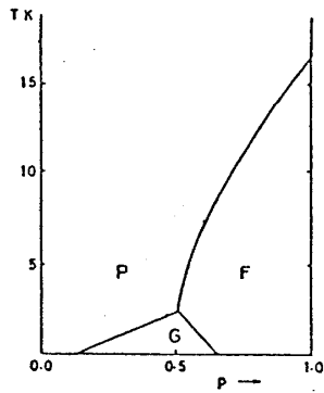
図4 Eu_pSr_{1-p}S の相図 15)
