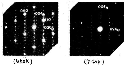
図2. 図1に於ける各領域からの電子回折図形
