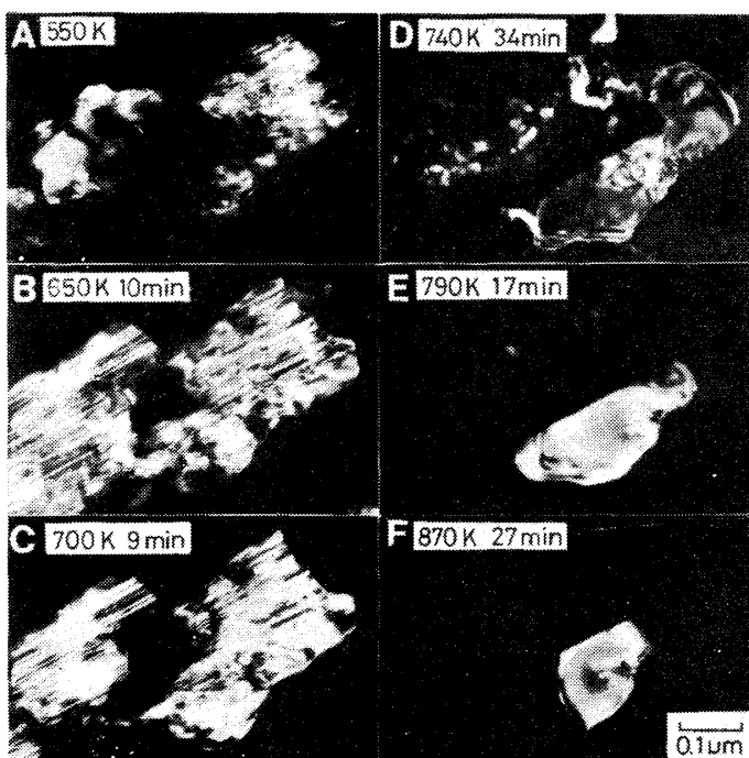
図1. 電顕“その場”観察による \theta' → \theta 粒子への構造変化セメントイトに於ける暗視野像
