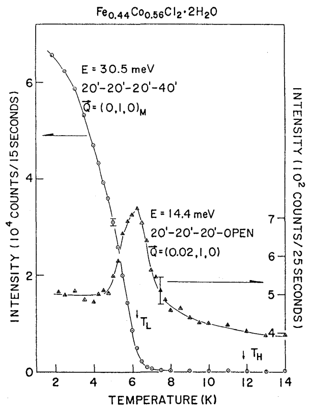
第4図 Fe_{0.44}Co_{0.56}Cl_2 \cdot 2H_2O の (0,1,0) 散乱強度の温度依存性
