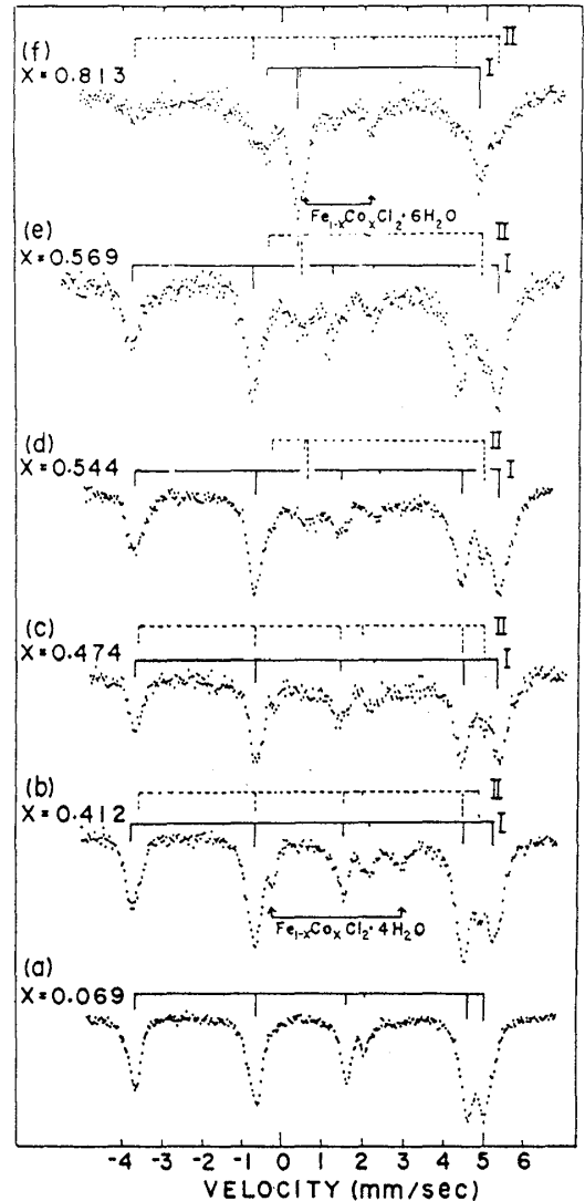
第6図 \text{Fe}_{(1-x)}\text{Co}_x\text{Cl}_2 \cdot 2\text{H}_2\text{O} の種々の濃度の単結晶で得られたメスbauerアスペクトル。測定温度 4.2\text{K} , \gamma 線は結晶のb軸に平行
