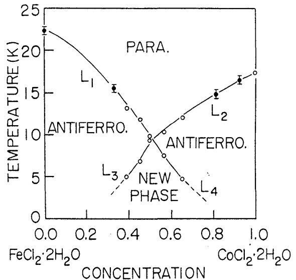
第3図 Fe_{(1-x)}Co_xCl_2 \cdot 2H_2O の濃度対転移温度の相図。○：比熱測定 ●：帯磁率測定より得られた転移点
