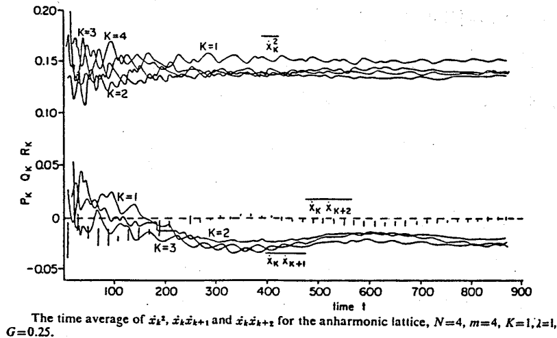
図1. 運動エネルギーと、速度の相関 両端固定、動きうる粒子の数4、 k は粒子の番号、( k=1, \dots, 4 )
