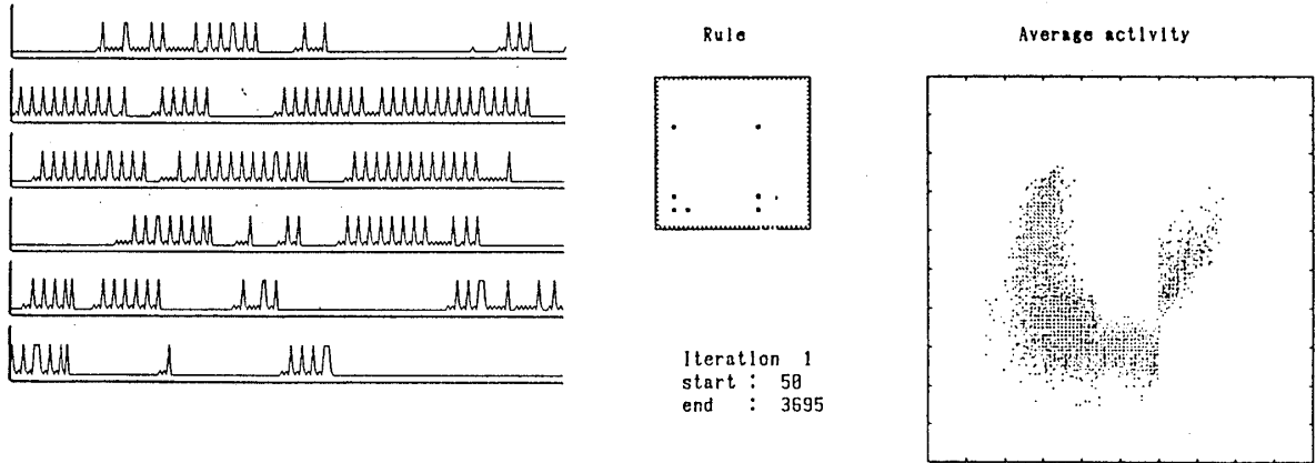
図2 インターミットルールダイナミクスの平均活動度のアトラクタ。左がルールのリターンマップ、右が平均活動度のリターンマップである。50 ステップまでの過渡期を除いて描いてある。
