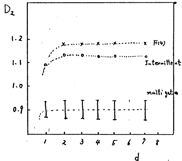
図4 いくつかのファジーアトラクタの相関次元。 F(4) 、インターミットtent、マルチゲートの3種類に対して、相関次元の埋め込みによる変化が描かれている。
