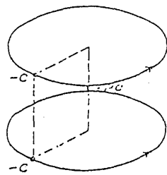
図 1: 1920 年代までに考えられたヘリウム原子の古典モデル [1] fig.1 から順番に Bohr, Langmuir, Landé, Langmuir のモデル
