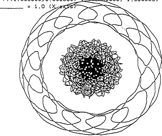
図 9: config.2: (r_1, v_1) = (3.0, 0.34) , T \approx 460 周期性のある形になった。ただし、 v_1 の走査では、上図からは連続的に変形できない。
