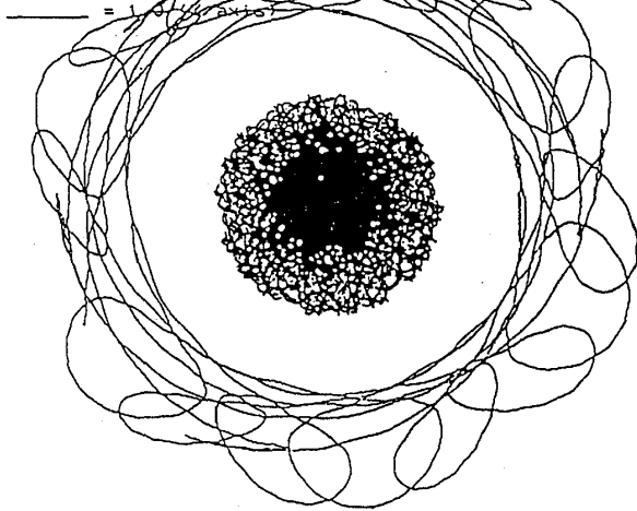
図 8: config.2: (r_1, v_1) = (3.0, 0.40) , T \approx 872 ループがかなり不規則になった
