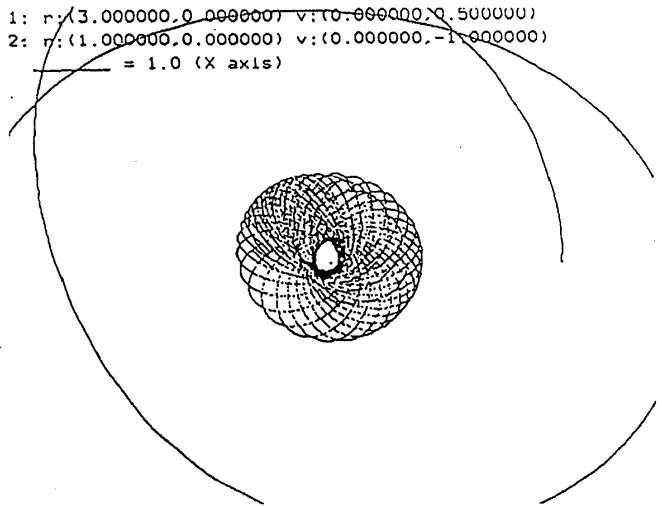
図 6: config.2: (r_1, v_1) = (3.0, 0.50) , T \approx 112 変形は見られない。
