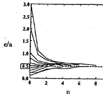
図5 b=d=0 の条件下で、様々な a, c, e の 組み合わせから出発した場合の e/a の 繰り込みによる変化
