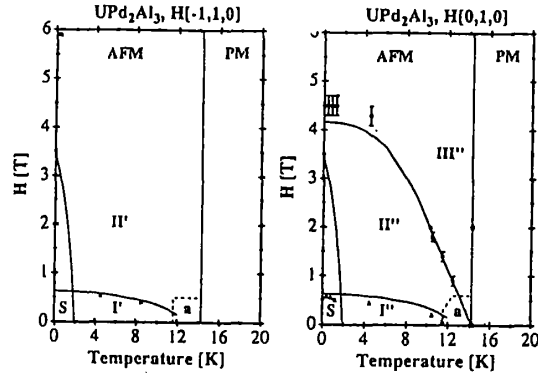
図7 磁気相図[4]
