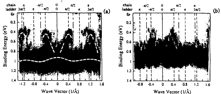
図2 実験から得られたSr x Ca 14-x Cu 24 O 41 (x=0,6)のバンド分散(図中の黒い部分)チェーンとラダーのブリルアンゾーンの周期(ka=0, π/2, π,...)を破線で示した。
