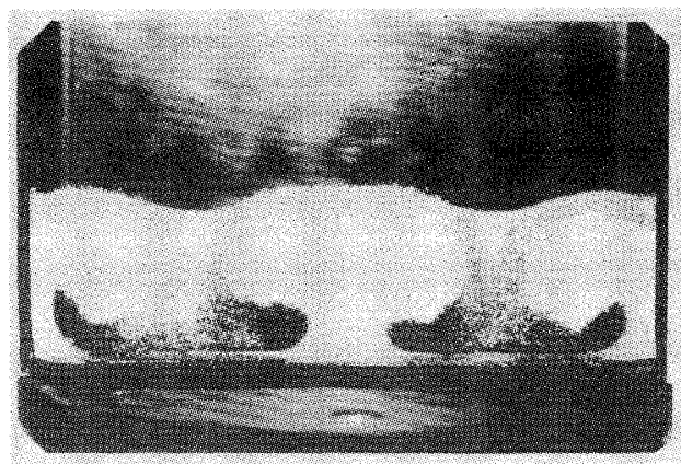
図3：粉体振動層に現れる対流ロール [8]
