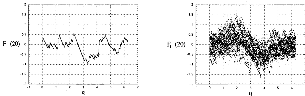
図 4: 実効的加速度 F_1(20)
