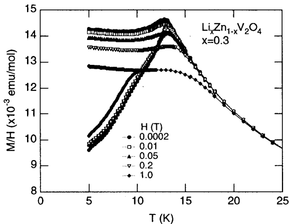
図2 : \text{Li}_{0.3}\text{Zn}_{0.7}\text{V}_2\text{O}_4 の直流磁化の磁場依存性。
