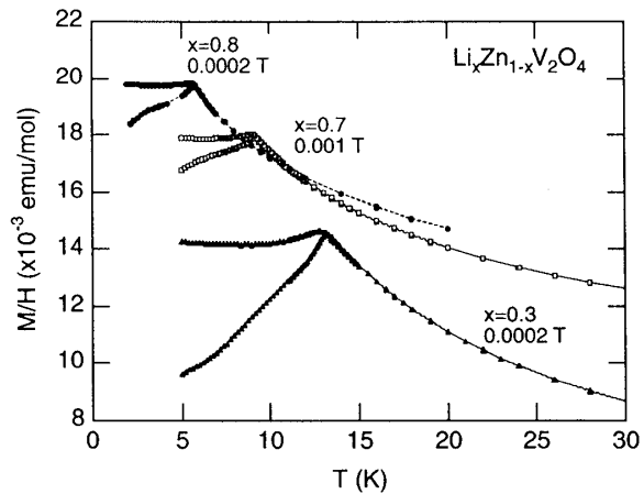
図1 : \text{Li}_x\text{Zn}_{1-x}\text{V}_2\text{O}_4 の弱磁場中での直流磁化。
