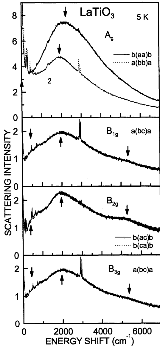
図 2: LaTiO 3 の 5K でのラマンスペクトル
