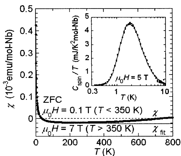
図 1: Y_2Nb_2O_7 の磁化率の温度変化。データは零磁場冷却 (ZFC) 後に測定したものを示した。挿入図に、磁場中における磁気比熱を示した。
