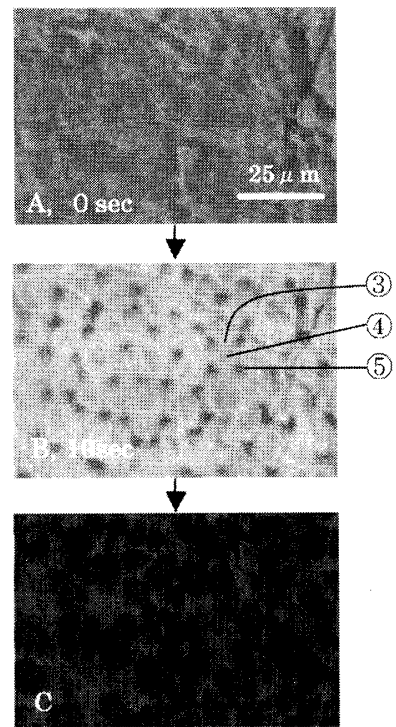
図4、A,B,C(右)：顕微鏡写真。A,B はそれぞれ図3の 0sec,10sec に対応している。B は3つの領域にわかれている(③,④,⑤)。また、温度変化を止めると暗い部分は徐々に統合していく(B→C)。
