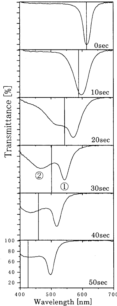
図3(左)：透過スペクトルの時間変化。図中の傍線は平衡位置でのピーク波長。先に進んでいるピーク②と遅れて進むピーク①に分かれている。
