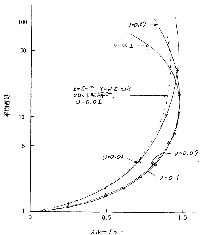
図2. スロットー遅延特性
