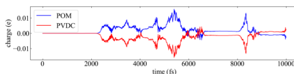
図：高分子の衝突と帯電量の時間変化の例。 Polyoxymethylene と polyvinylidene chloride
