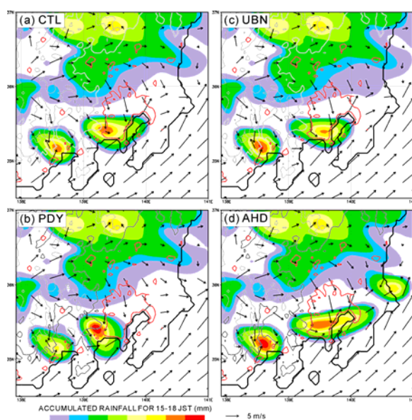
図 1 : CReSiBUC で計算された (a)CTL、(b)PDY、(c)UBN、(d)AHD による 3 時間積算降水量分布。赤線で囲まれた領域は、土地利用分布データにおいて感度実験の際にデータ操作を行った都市領域を示す。
