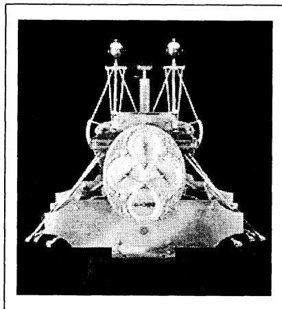
図2 H-1型クロノメータ
