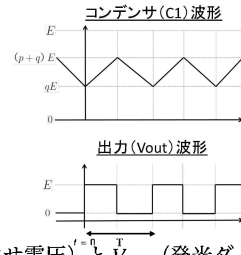
図6: V (コンデンサ電圧)と V_{out} (発光ダイオード出力)の回路特性
