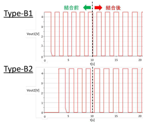
図 11: 出力波形 ( t = 10[s] において結合開始)
