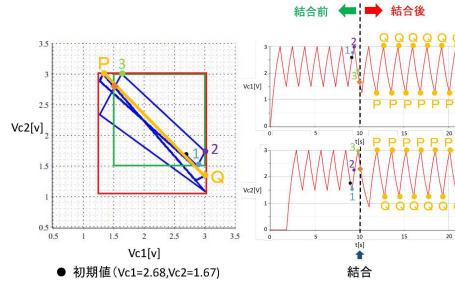
図 10: Type-A · Type-A 結合における相図
