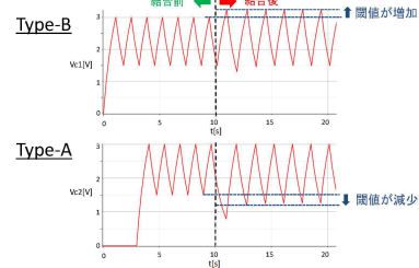
図 15: コンデンサ波形 ( t = 10[s] において結合開始)
