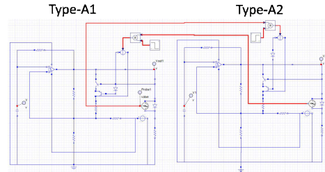
図 7: MapleSim での TypeA・TypeA の結合モデル
