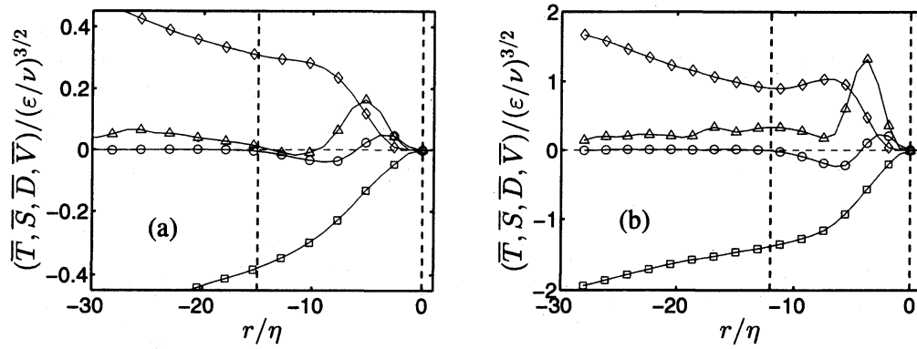
図 5: BL2 における乱れ渦度の強さ \phi の収支項の r 軸上の条件付き平均分布. (a) 境界面が平均位置 x_2 = 0.9\delta より壁に近い場合, (b) 壁から遠い場合. \triangle, \bar{T} ; \diamond, \bar{S} ; \square, \bar{D} ; \circ, \bar{V} . 縦の破線は粘性拡散がはたらくおよその範囲を示す.
