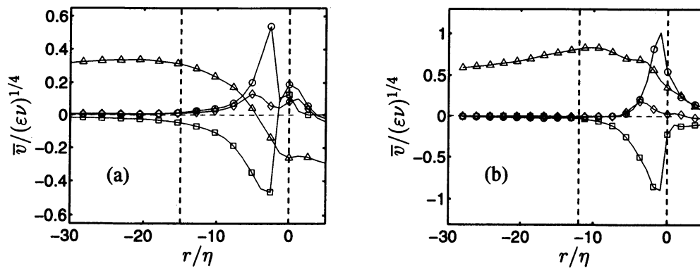
図 6: BL2 における仮想速度 v への T, S, D, V からの寄与の条件付き平均分布. (a) 境界面が平均より壁に近い場合, (b) 遠い場合. \triangle , -T/\nabla\phi ; \diamond , -S/\nabla\phi ; \square , -D/\nabla\phi ; \circ , -V/\nabla\phi . 縦の破線は粘性拡散がはたらくおおよその範囲を示す.
