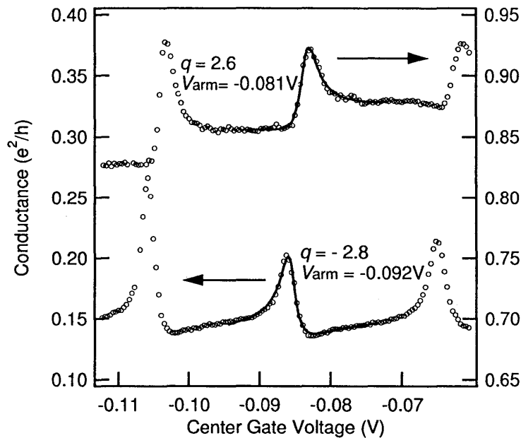
図 5.8: q の符号が反転する Fano ピーク。離散準位と連続準位との位相の差が \pi 程度あるものと考えられる。実線は q を実数としてフィッティングしたもの。
