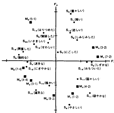
図5 ALSCAL-4 モデルによる分析結果
