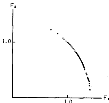
図4 個人モードの重み係数 (PARAFAC)
