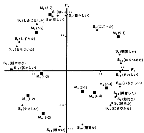
図 2 因子分析法による分析結果
