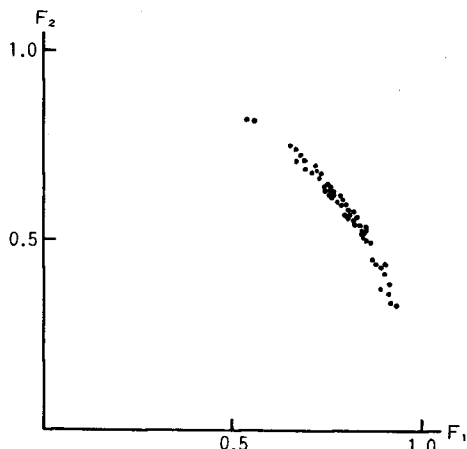
図6 個人モードの重み係数 (ALSCAL-4)
