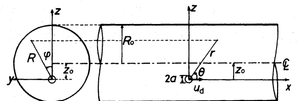
図5. 振動型ホアズイユ流
