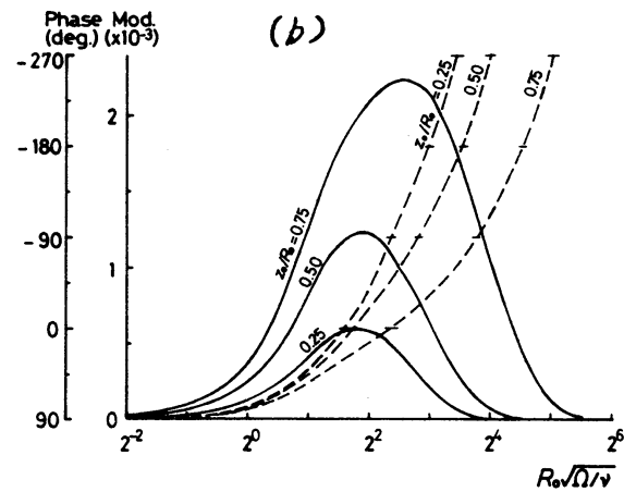
図7. 振動型ポアズエ流の球の角速度. (a) 2\Omega/(-2R_0) の絶対値と位相角, (b) その相対誤差 (2\Omega - \omega_y)/(-2R_0)
