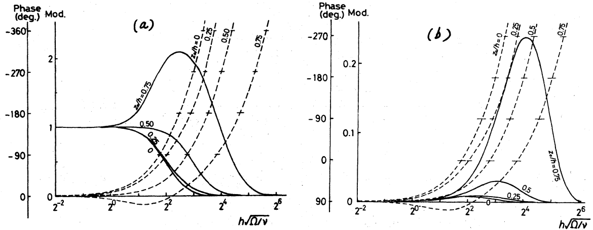
図4. 振動型ジェット流中での球形粒子の回転角速度 2h\Omega/U (a) と、乱れのない渦度場に対する相対誤差 (2\Omega - \omega_y)h/U (b). いずれも \gamma = 1/15 , a/h = 0.1 とする。
