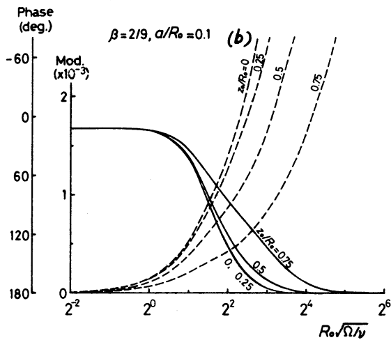
図6. 振動型ポアズエ流の球の移動速度. (a) u/(c-2R_0^2) の絶対値と位相角, (b) その相対誤差 (u - u_0)/(c-2R_0^2)
