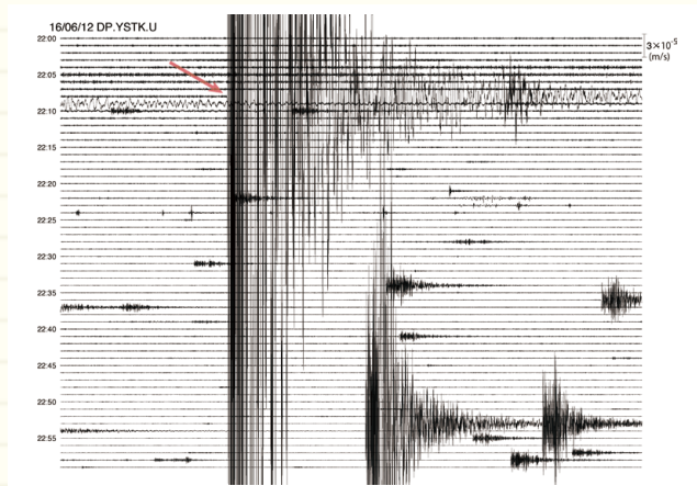
図1 熊本県八代市に設置した臨時観測点で観測された2016年6月12日22時台の波形記録(上下動成分)。22時08分に最大震度5弱を観測した地震(赤矢印)や、その後に続いたいくつかの余震の記録が収録できている。
